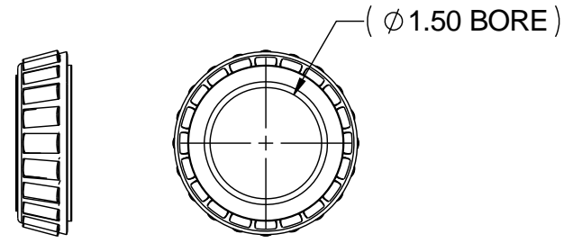
3X X000-4300-J0408 CONE
