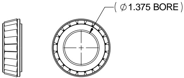
1X X000-4300-J0411CONE
